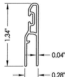
15 SILL RISER
